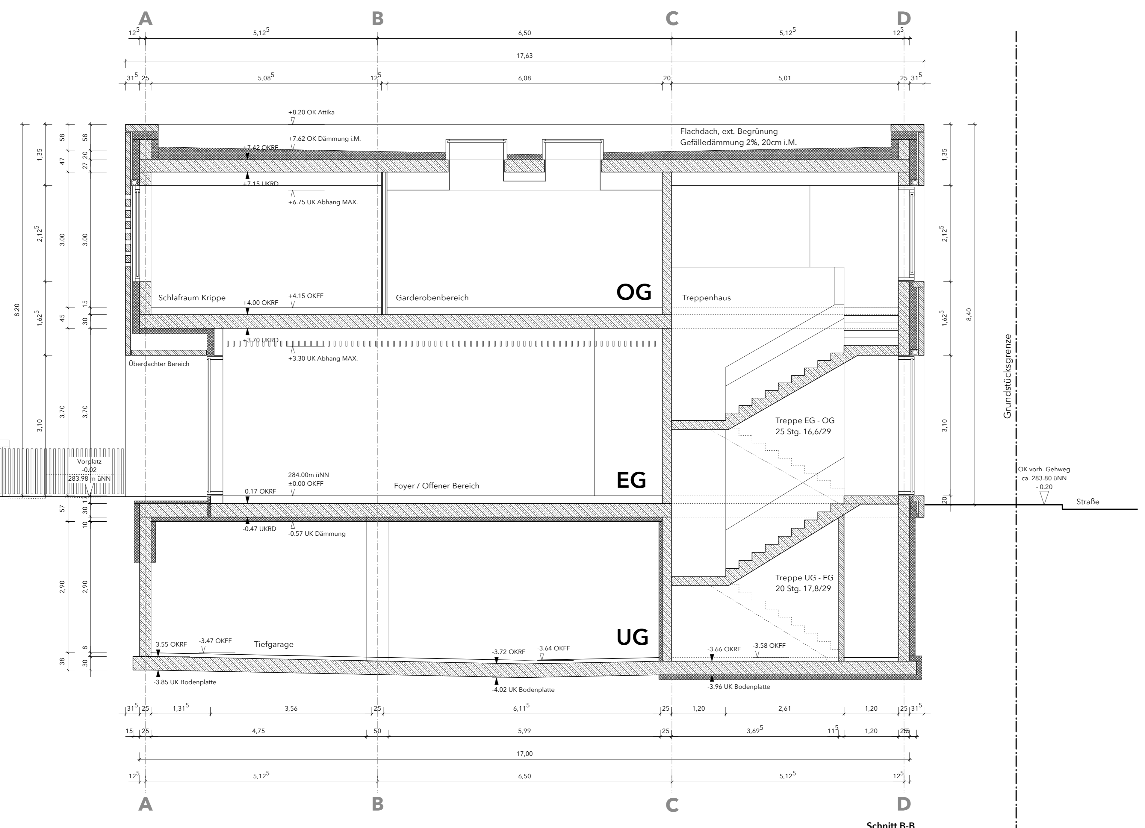
Schnitt B-B
