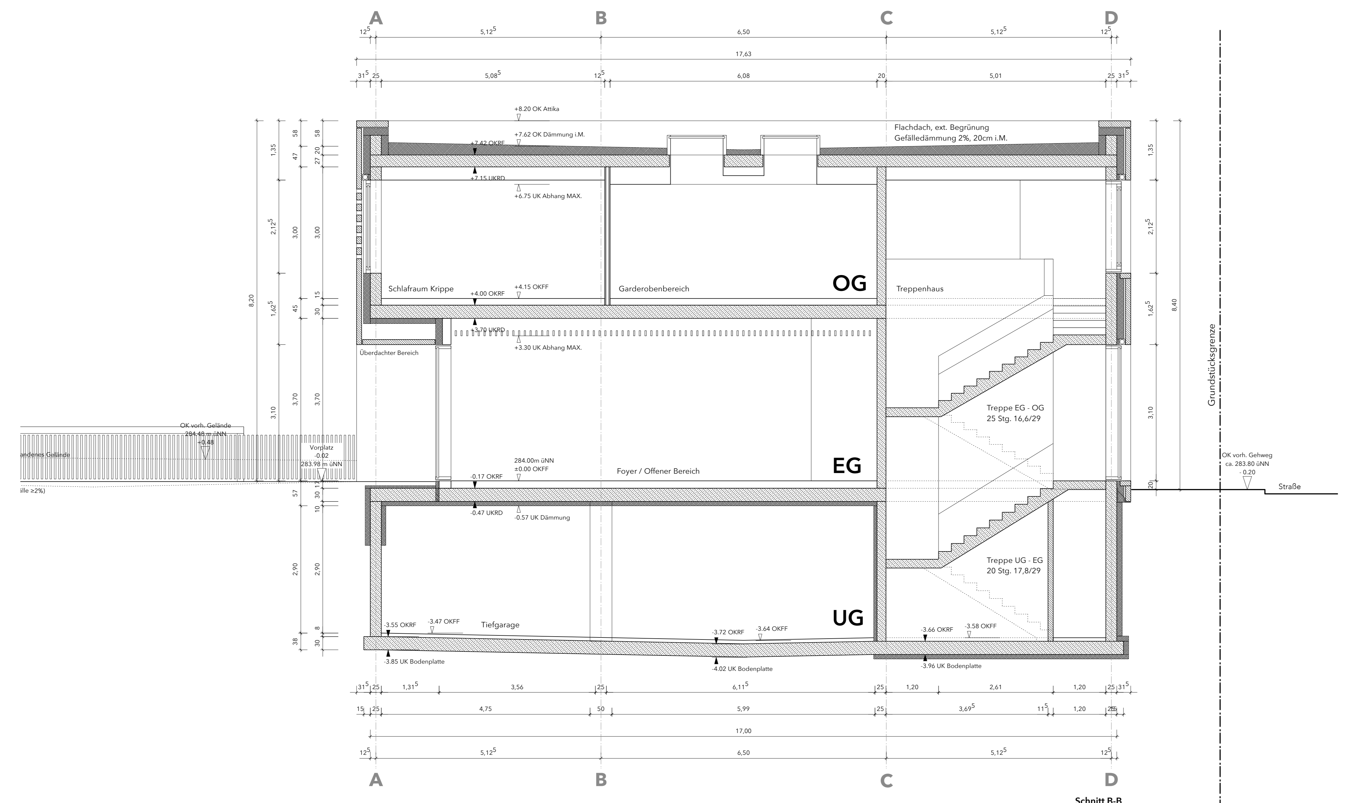
Schnitt B-B
