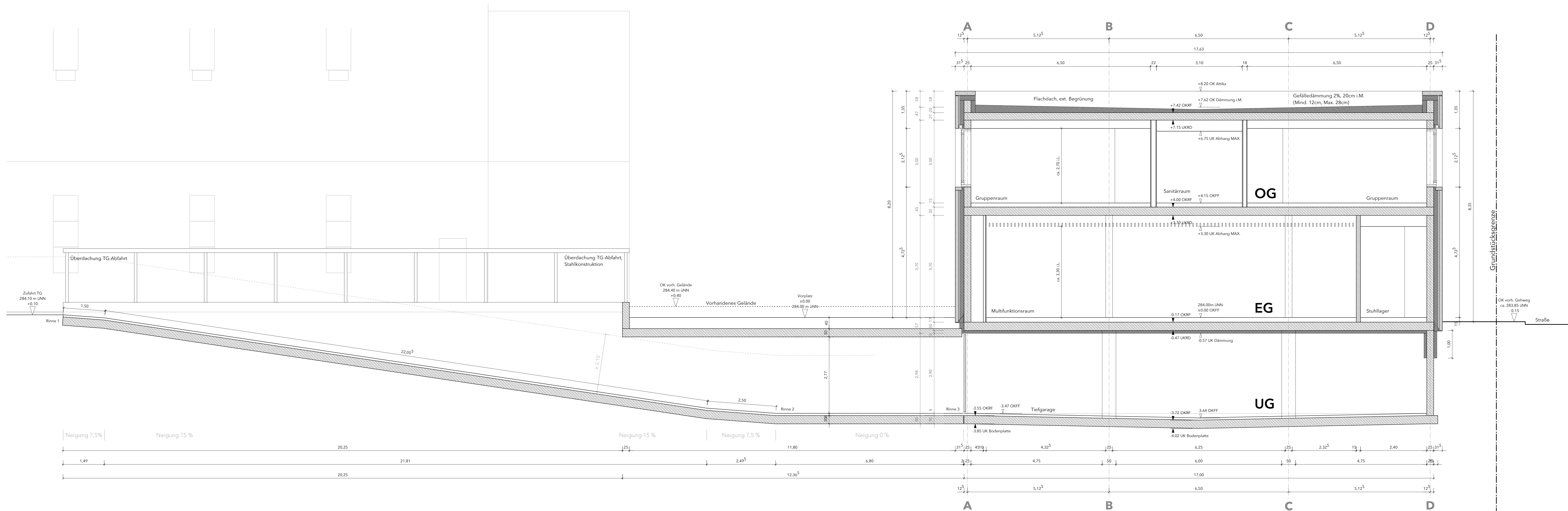
Schnitt A-A
